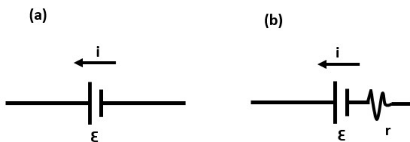
Figura 7: (a) Gerador ideal, não apresenta perdas internas. (b) Gerador real, apresenta perdas internas. Sua resistência interna é dada por r e a força eletromotriz \mathcal{E} é maior que a tensão externa entregue a um circuito. Fonte: Autor.
