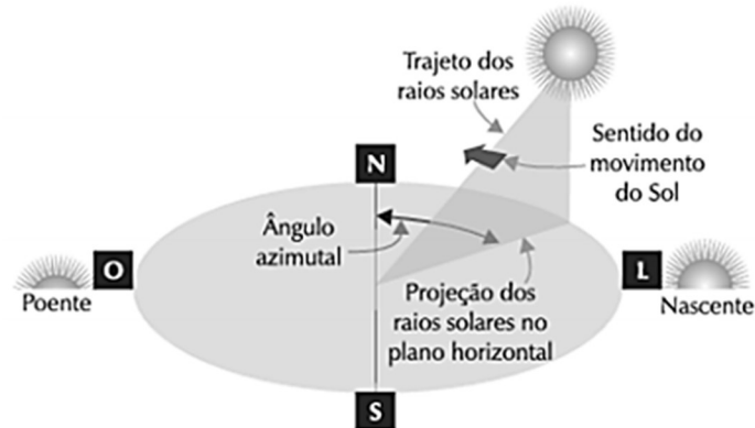
Figura 14: Ângulo azimutal
