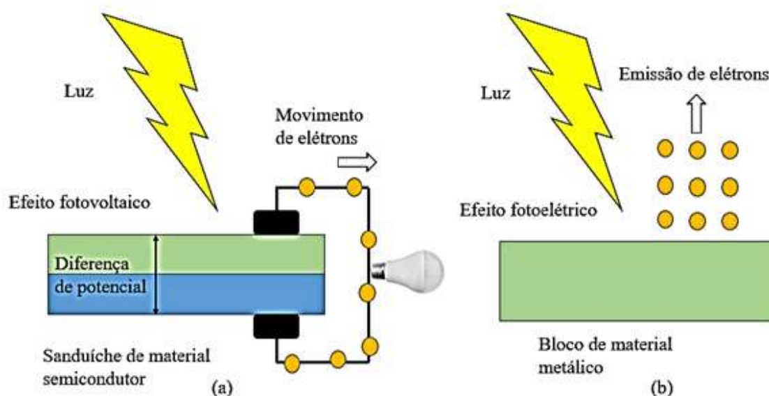
Figura 10: Efeito fotovoltaico (a) e efeito fotoelétrico (b).
